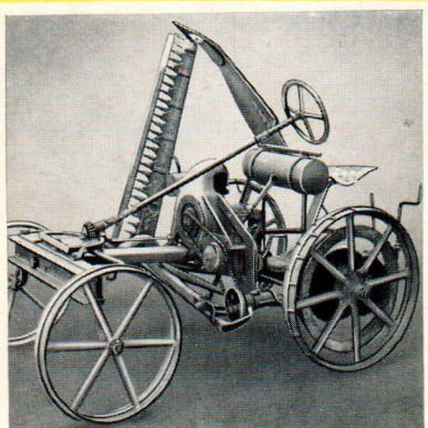
Der erste Kramer-Kleinschlepper mit Motormäher 1925
