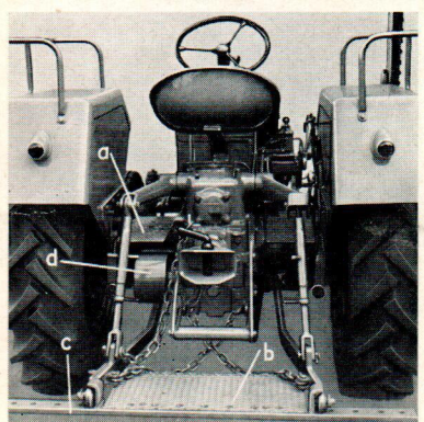
Zentralhydraulik mit Dreipunktaufhängung a = große Fußbleche b = Ladepritsche c = breite Ackerschiene d = Riemenscheibe
