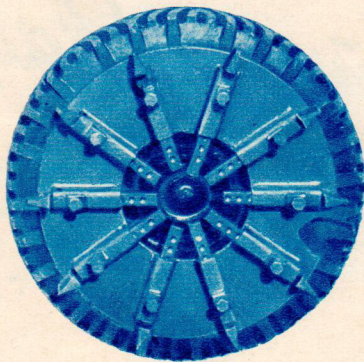
Greiferrad mit eingezogenen Greifern
